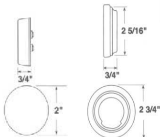
AJOUTER 1/4" POUR L'INSTALLATION ADD 1/4" FOR INSTALLATION
